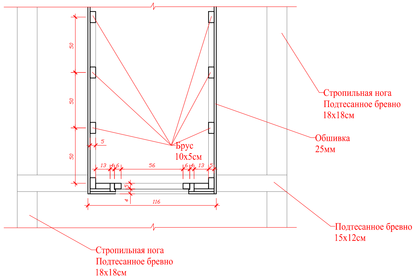
Разрез 2-2. М 1:20
