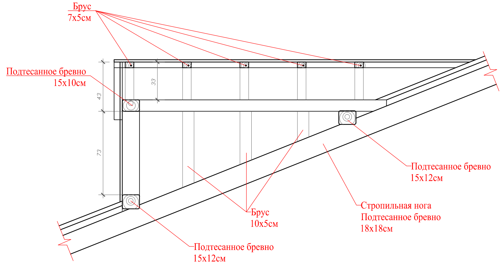
Разрез 1-1. М 1:20
